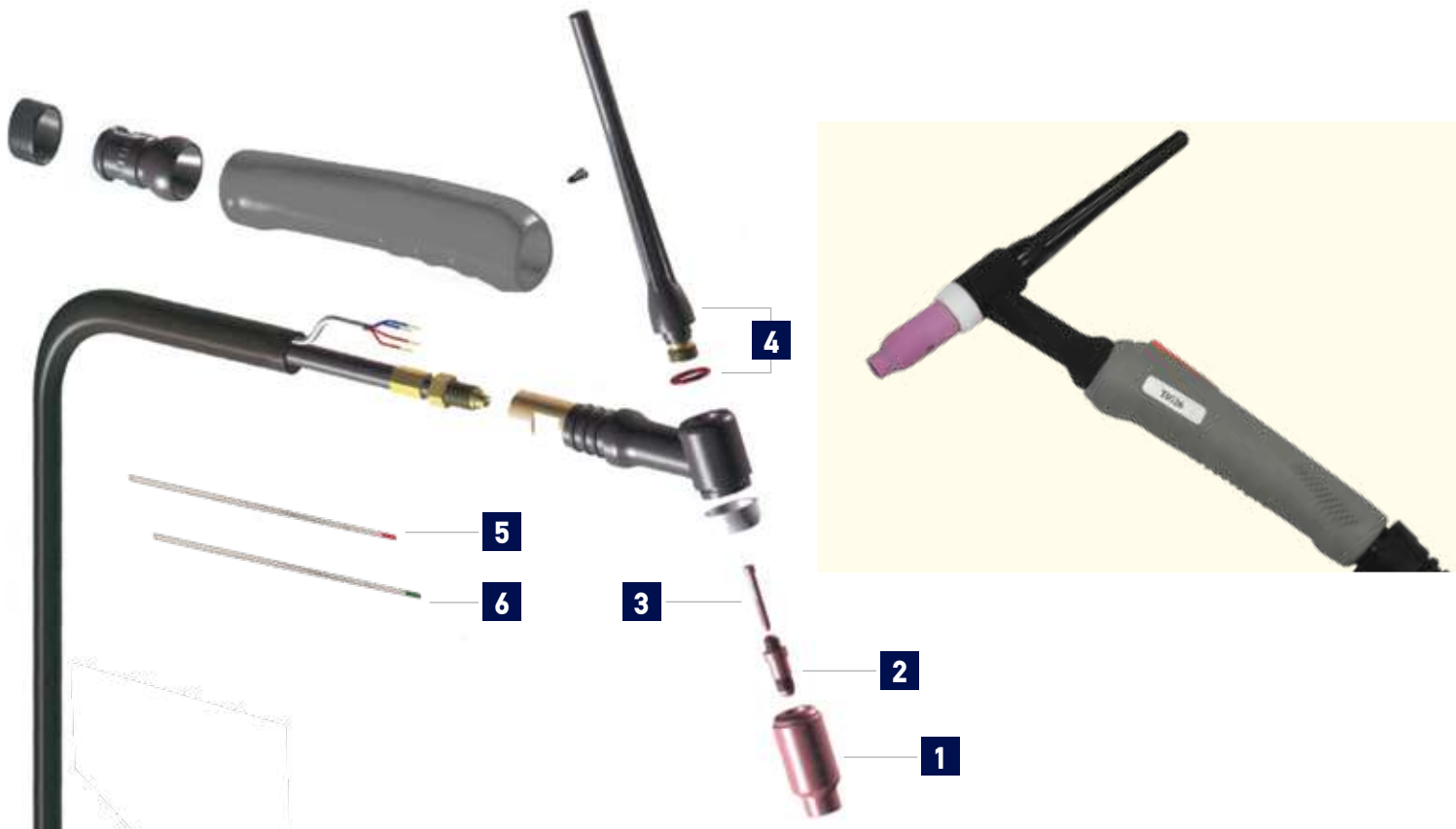
ΤΣΙΜΠΙΔΑ SR 26
