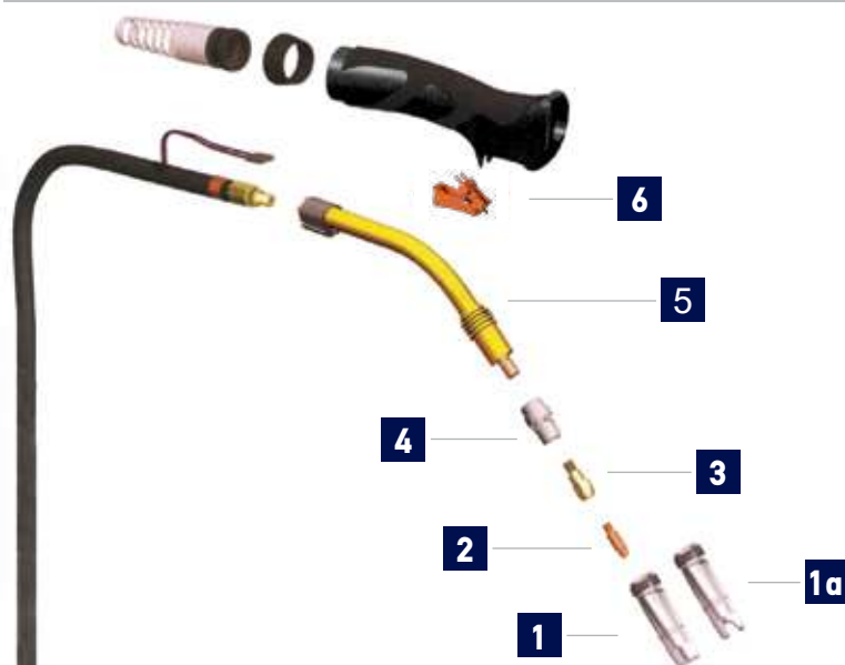
ΤΣΙΜΠΙΔΑ MIG 36
