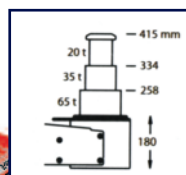
N20-3C 65 ton. max. 3 εμβόλων
