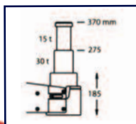
N15-2L 30 ton. max. 2 εμβόλων
