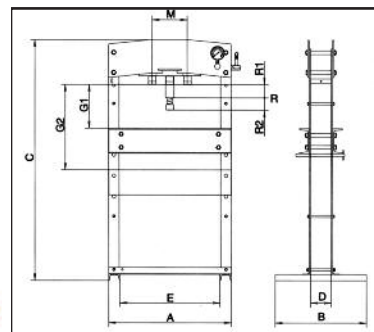
KCK - 30A Δαπέδου 30 ton.
